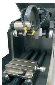
Détail des guidages du chariot avec déplacement latéral TRA 032. Course 80 mm Vernier 0,05 mm
