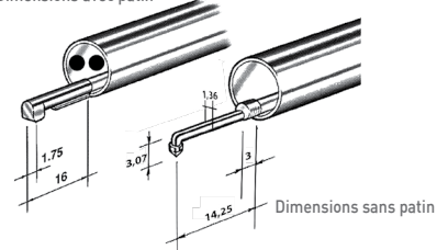
Dimensions avec patin
