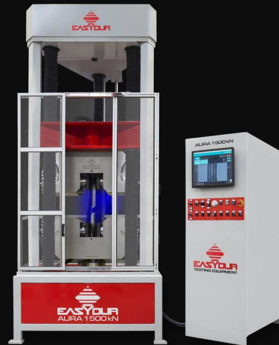
AURA TENSILE Jusqu'à 1500 kN
