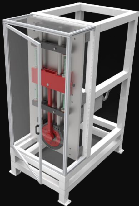
SYSTÈME VERTICAL FAT 600 MANIVELLE ET TIGE
